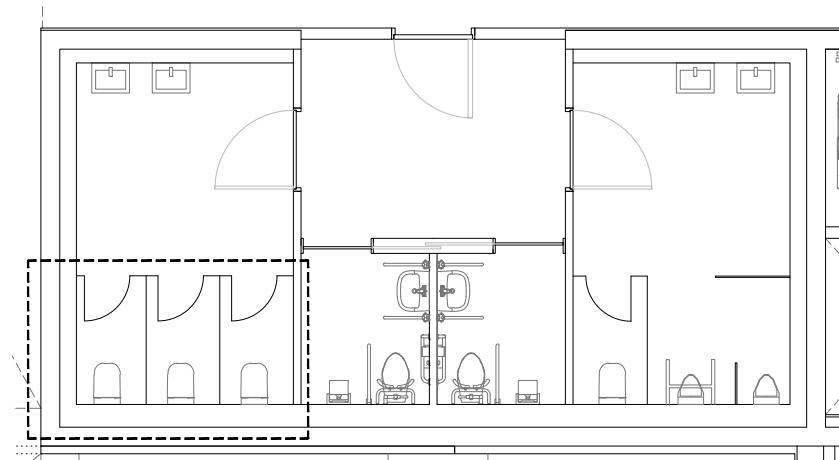
EXAMPLE: F2 EXPOSITION WC CORE 1:100
